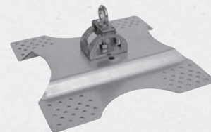
Punto d'ancoraggio studiato per strutture fragili, a completamento della linea vita in classe C Securope®. In caso di caduta la parte superiore dell'ancoraggio si abbatte, riducendo gli sforzi trasmessi alla struttura.
